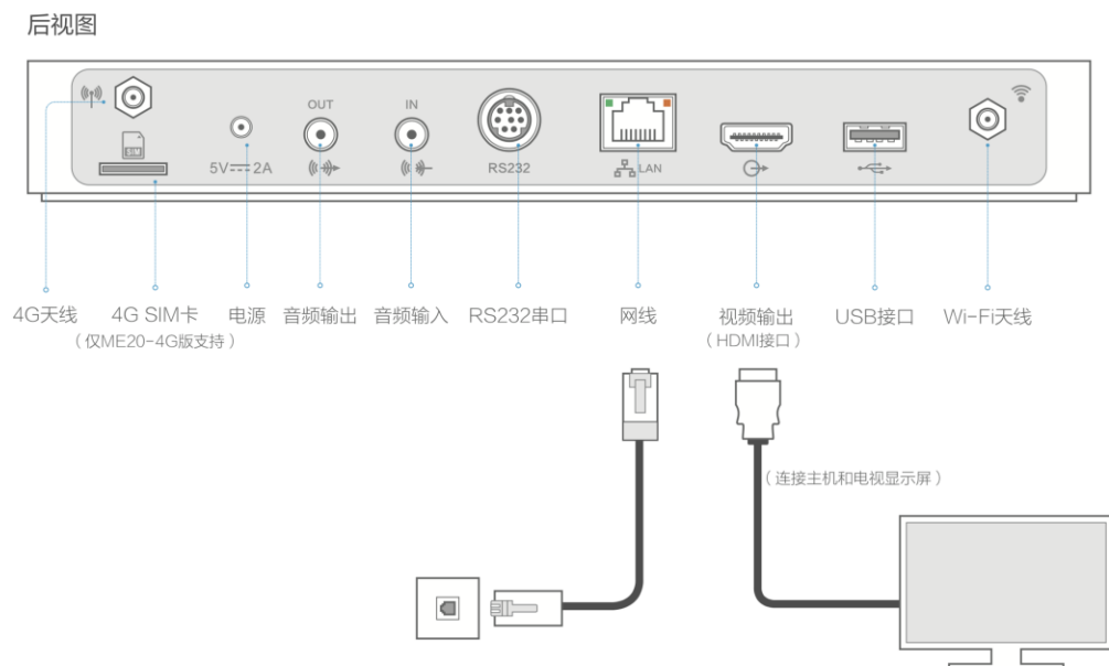
图 1-1 线缆连接示意图
