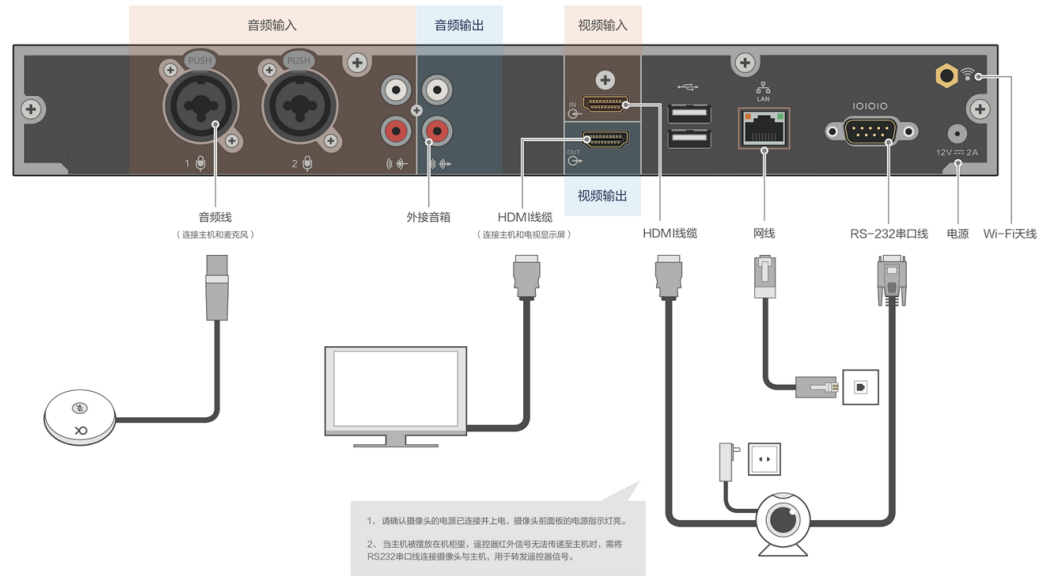
图 3-1 线缆连接示意图
