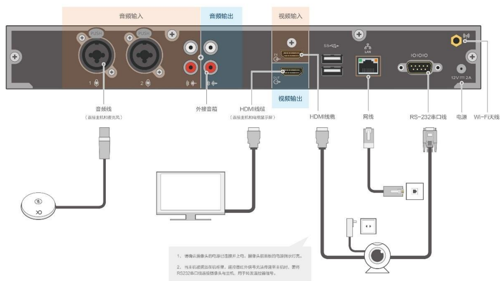
图 1-1 线缆连接示意图
